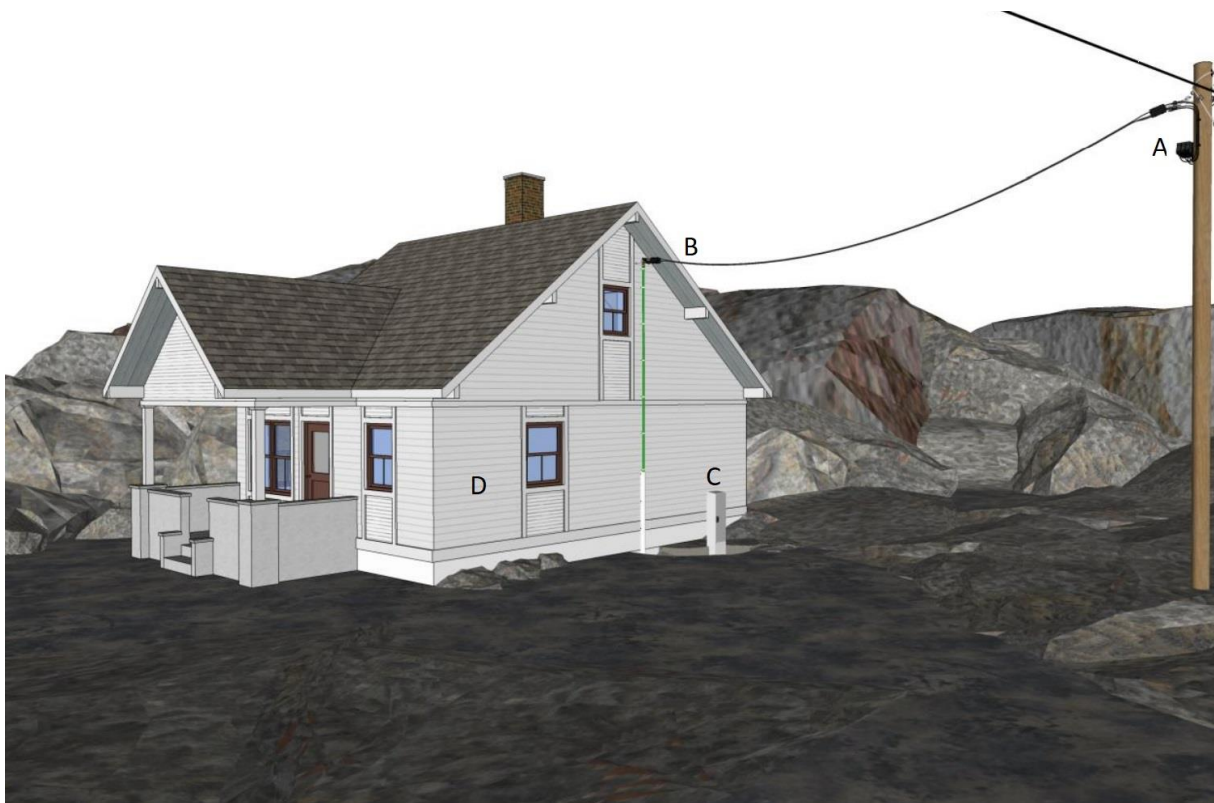
Figur 5 - RT11211 "Installasjonsendring i forbindelse med omgjøring fra 1-fase til 3-fase luftnett" (hentet fra RENblad 4100)
