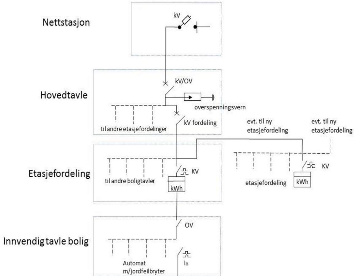
Figur 4 - Enlinjeskjema "blokk prinsipp" tavle og etasjefordelere (fra RENblad 4100)
