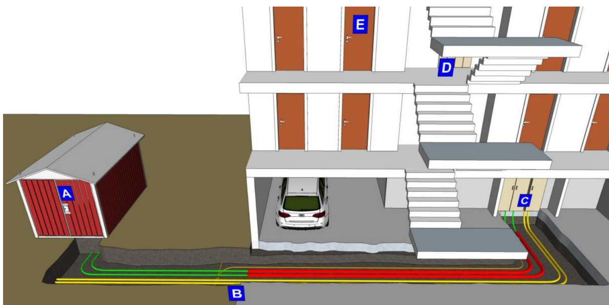
Figur 3 - RT11051 "blokk prinsipp" tavle og etasjefordelere (figur hentet fra RENblad 4100)
