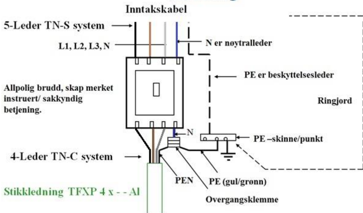
Figur 6 - Splitting av PEN leder i fordeling
